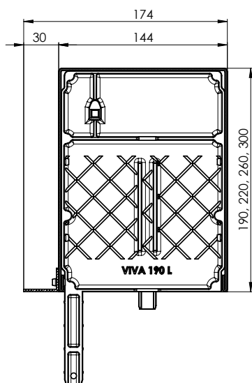
Řez přiznaného boxu VIVA + P 020/03, P 080/03, P 081/03
