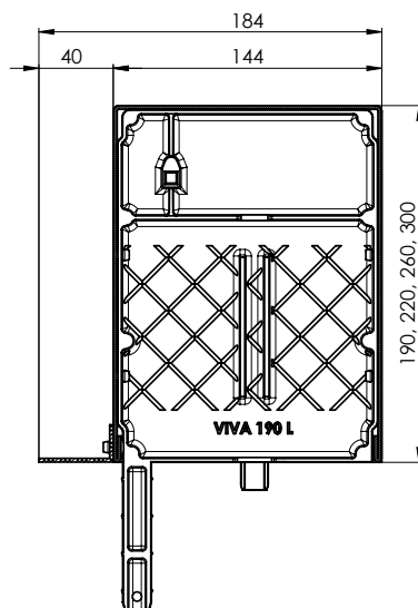
Řez přiznaného boxu VIVA + P 020/04, P 080/04, P 081/04
