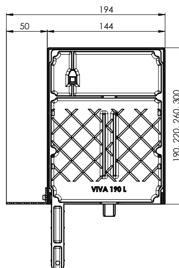
Řez přiznaného boxu VIVA + P 020/05, P 080/05, P 081/05
