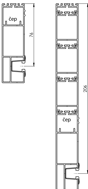
Základní profil P 020 Maximální možné rozšíření základního profilu P 020
