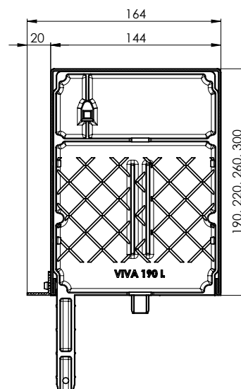
Řez přiznaného boxu VIVA + P 020/02, P 080/02, P 081/02
