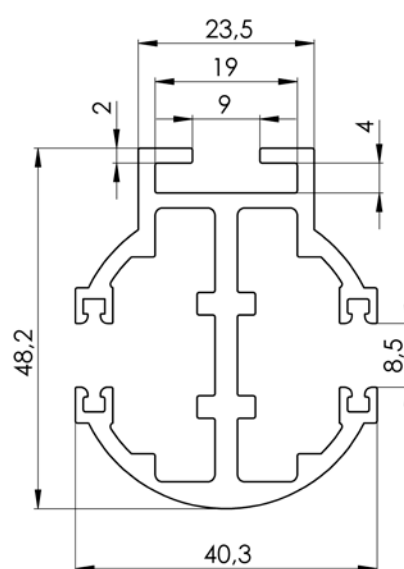
Kruhová vodicí lišta dvojitá P 017/7 (7-302155)
