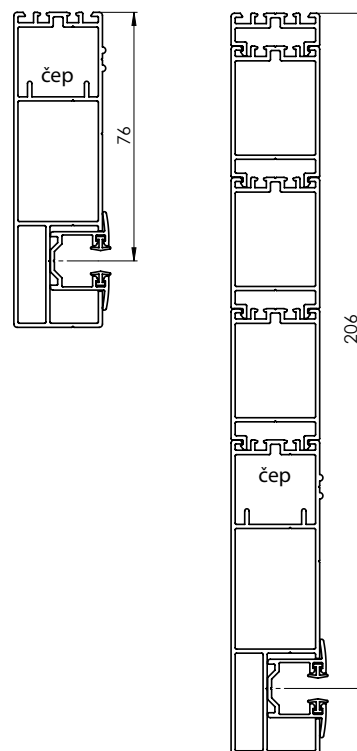
Základní profil P 081 Maximální možné rozšíření základního profilu P 081
