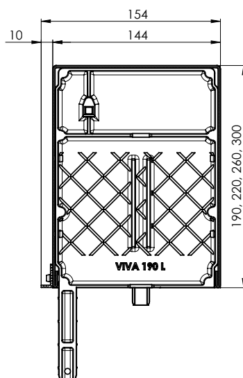
Řez přiznaného boxu VIVA + P 020/01, P 080/01, P 081/01
