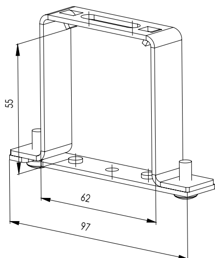
Věšák horního profilu Fe P 002 (2-00038) (pro horní profil 56x58) Tento typ věšáku je dodáván vždy bez nástříku.
