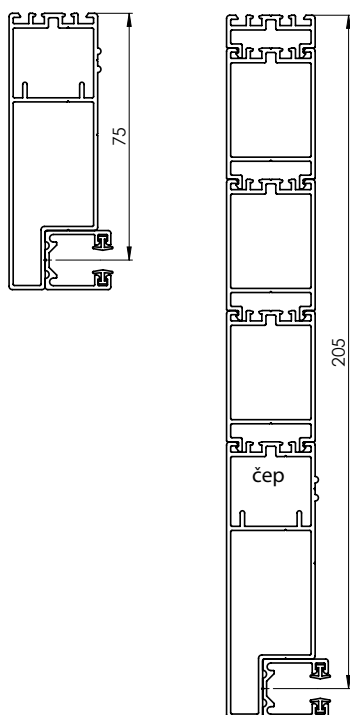
Základní profil P 080 Maximální možné rozšíření základního profilu P 080
